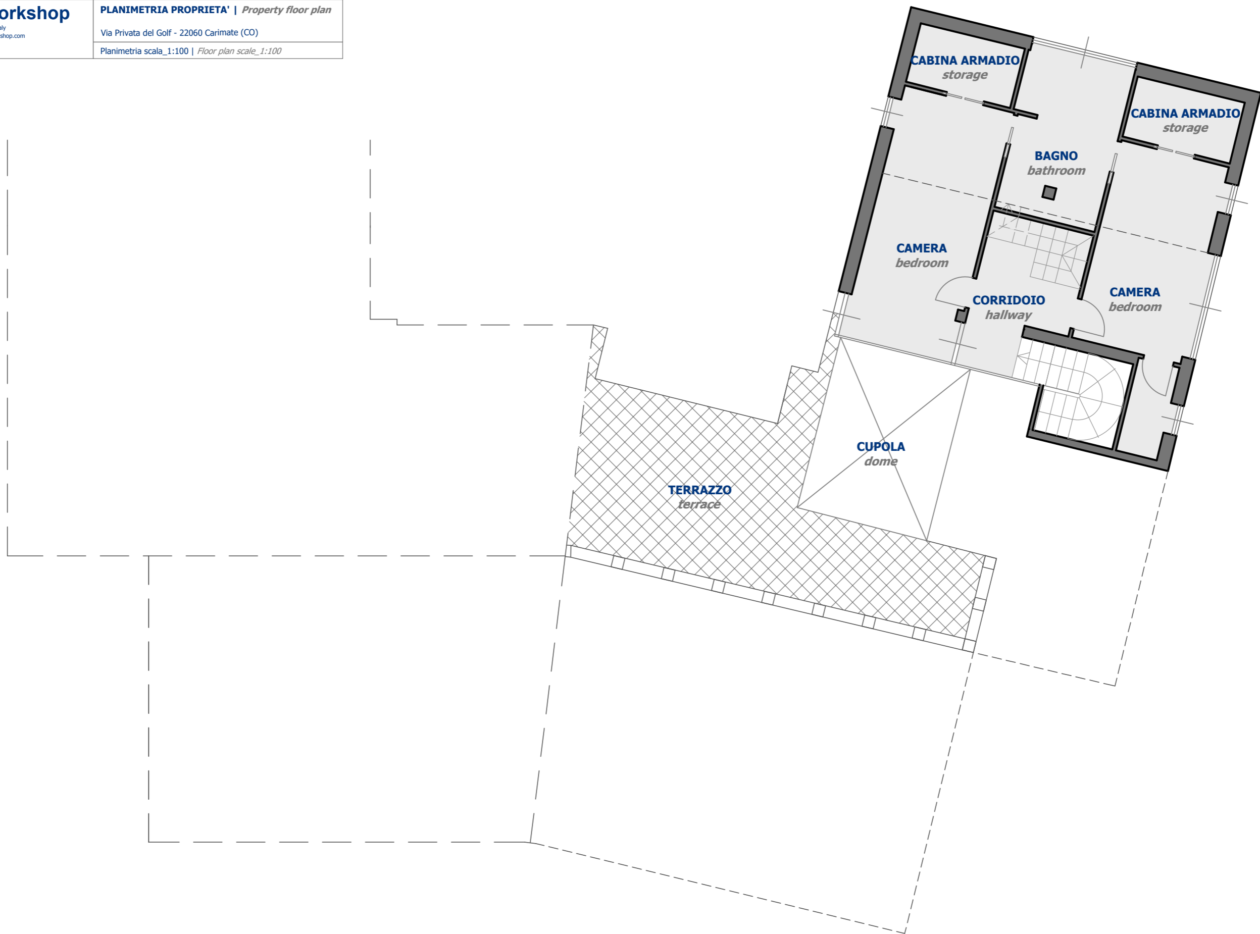
Planimetria Piano Secondo
